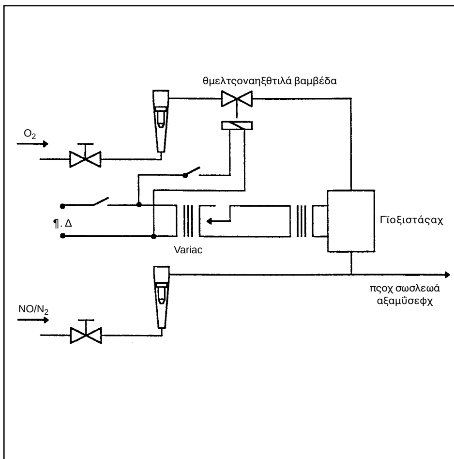
Σχηματική διάταξη ελέγχου αποδόσεως μετατροπέα \text{NO}_2
